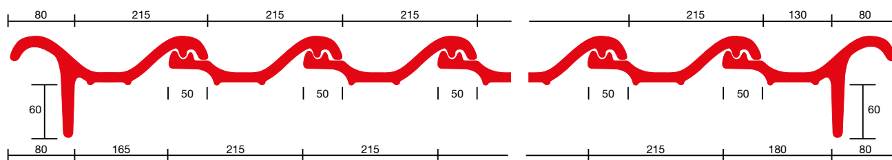
Dekkende breedte linker gevelpan 215 mm.
